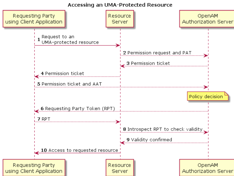
Figure 15.5. OpenAM in UMA RPT Token Flow
